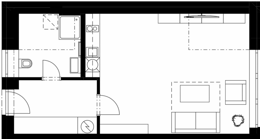
Půdorys B4
